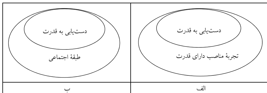
نمودار ۱. مفهوم‌سازی شرط لازم از طریق تئوری مجموعه‌ها
