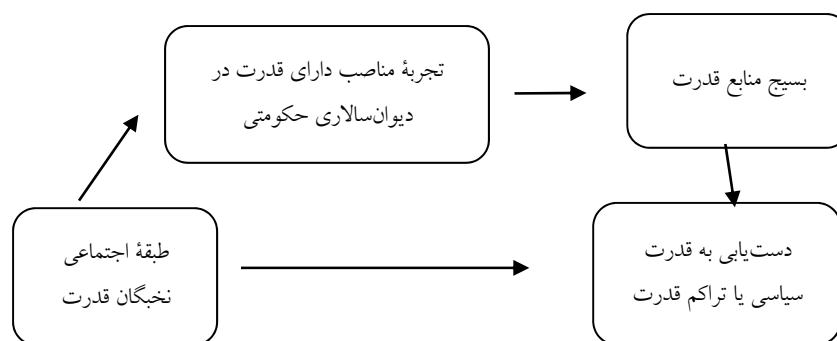
مدل تئوریک ۱
